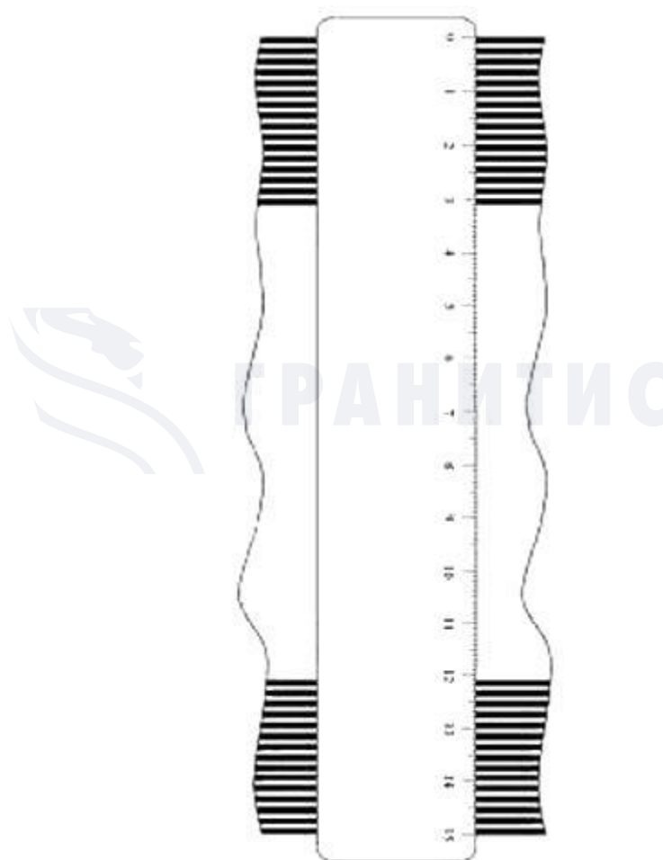
Рисунок А.1 - Измеритель профиля
